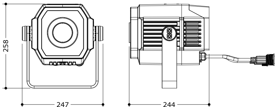
Disegno tecnico
