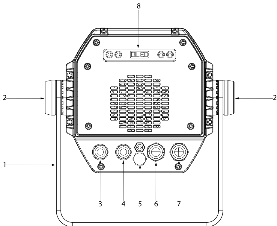
Pannello Posteriore
